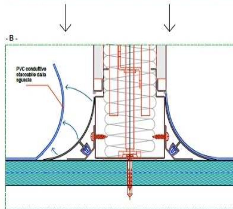
PVC AUTOPOSANTE A SECCO IN PIASTRE TERMOSALDABILE CONDUTTIVO O STATICO DISSIPATIVO SPESSORE 4mm
