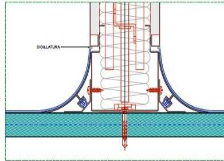
SEZIONE DETTAGLIO ATTACCO PARETE - PAVIMENTO IN PVC -A-
